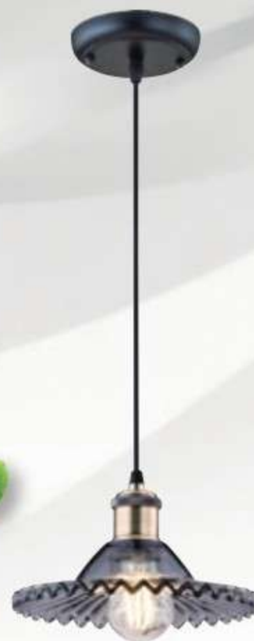
SH-23666 2800 W220mm H130mm 線長1000mm E27x1 另計 鋼材烤漆 鋁製品電鍍 煙灰色玻璃
