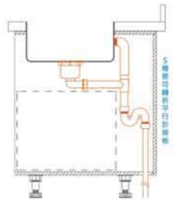
◎ 櫃體安裝示意圖
